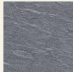
岩盤柄(25)
